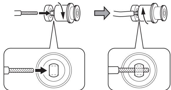
Sección transversal
